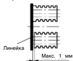
Рис. 5 Выверка шкивов ременной передачи
