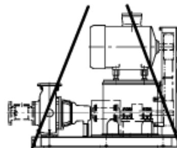
Рис. 2c Транспортировка насосного агрегата в сборе (тип установки 3Н с редуктором)
