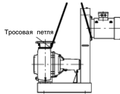
Рис. 2a Транспортировка насосного агрегата в сборе (тип установки 3Н)
